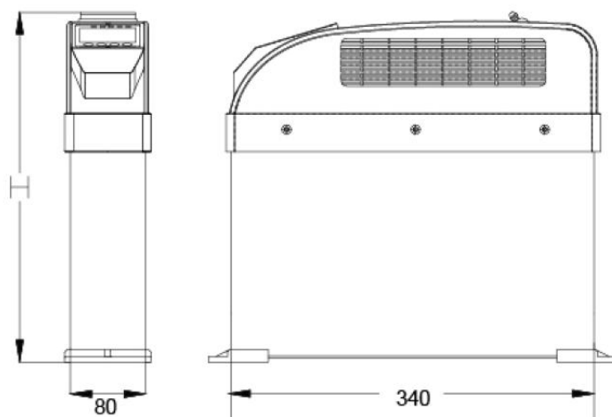
图 50 外形尺寸图
