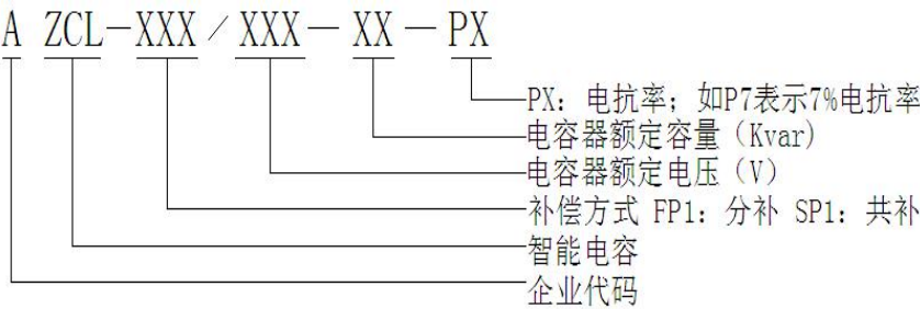
图 56 型号说明
