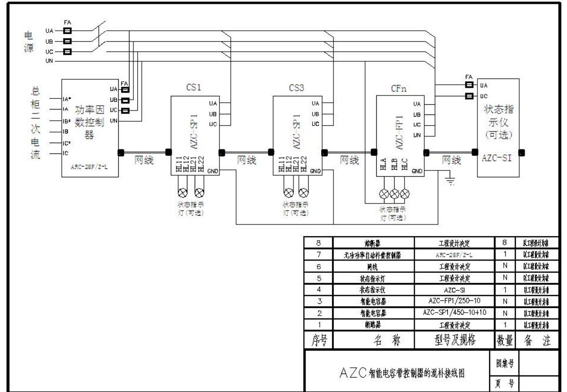
图 55 带无功补偿控制器的混补接线
