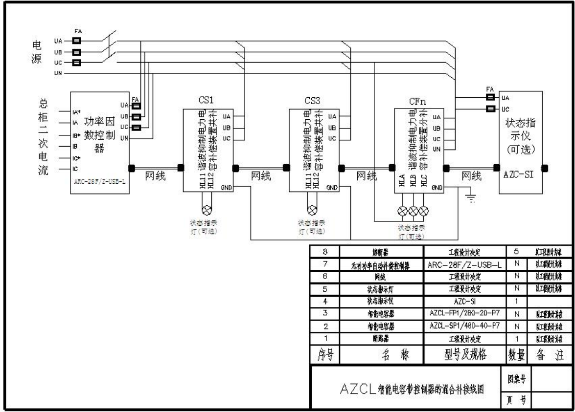
图 99 带无功补偿控制器的混补接线图
