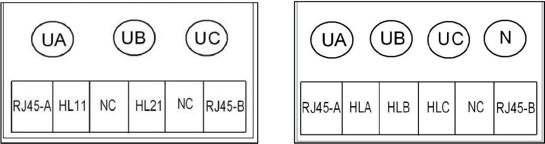
图 95 接线端子图
