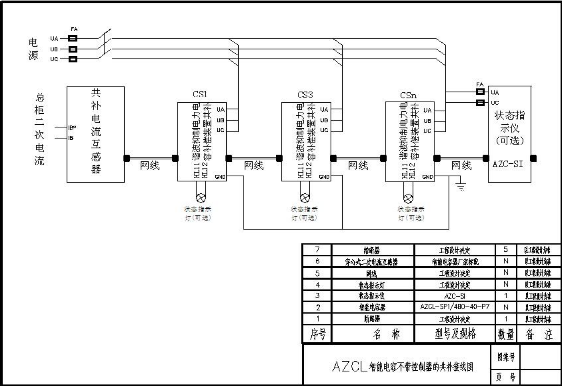
图 96 不带无功补偿控制器的共补接线
