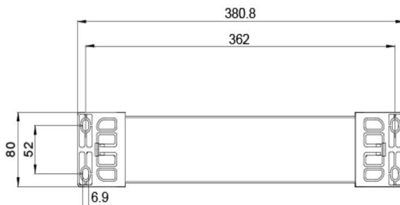
图 51 安装尺寸图
