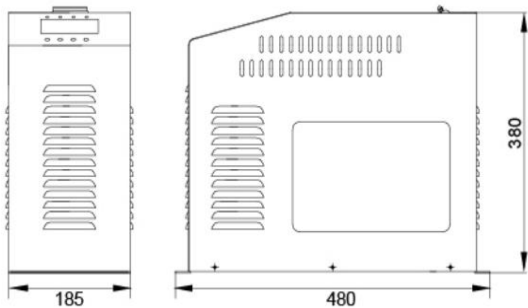
图 94 外形尺寸图
