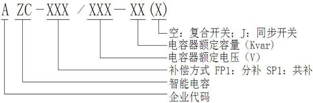
图 1 型号说明
