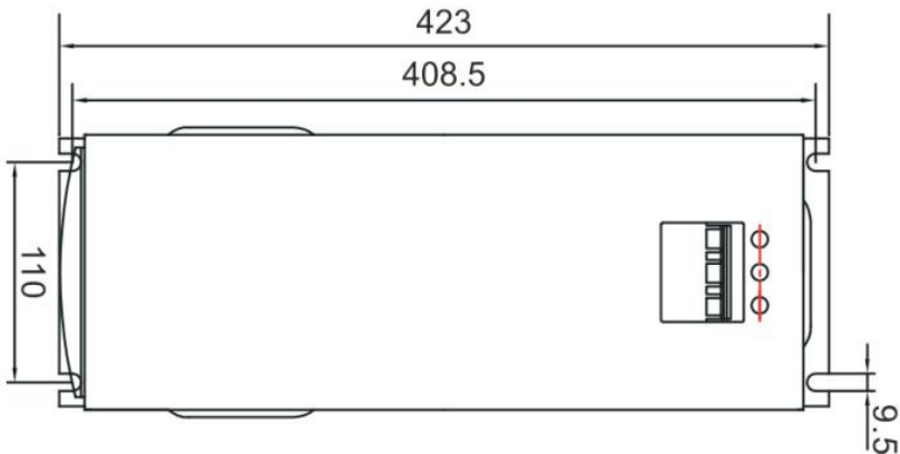
图 131 安装尺寸图
