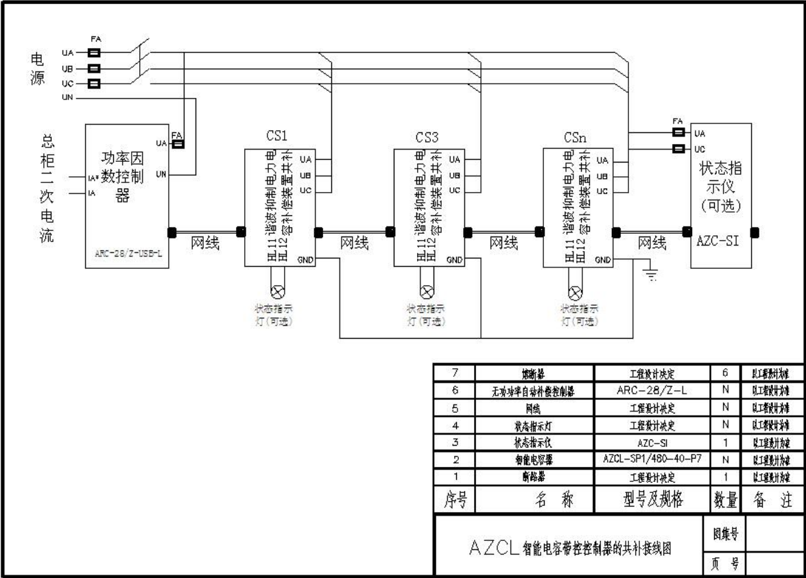
图 98 带无功补偿控制器的共补接线图
