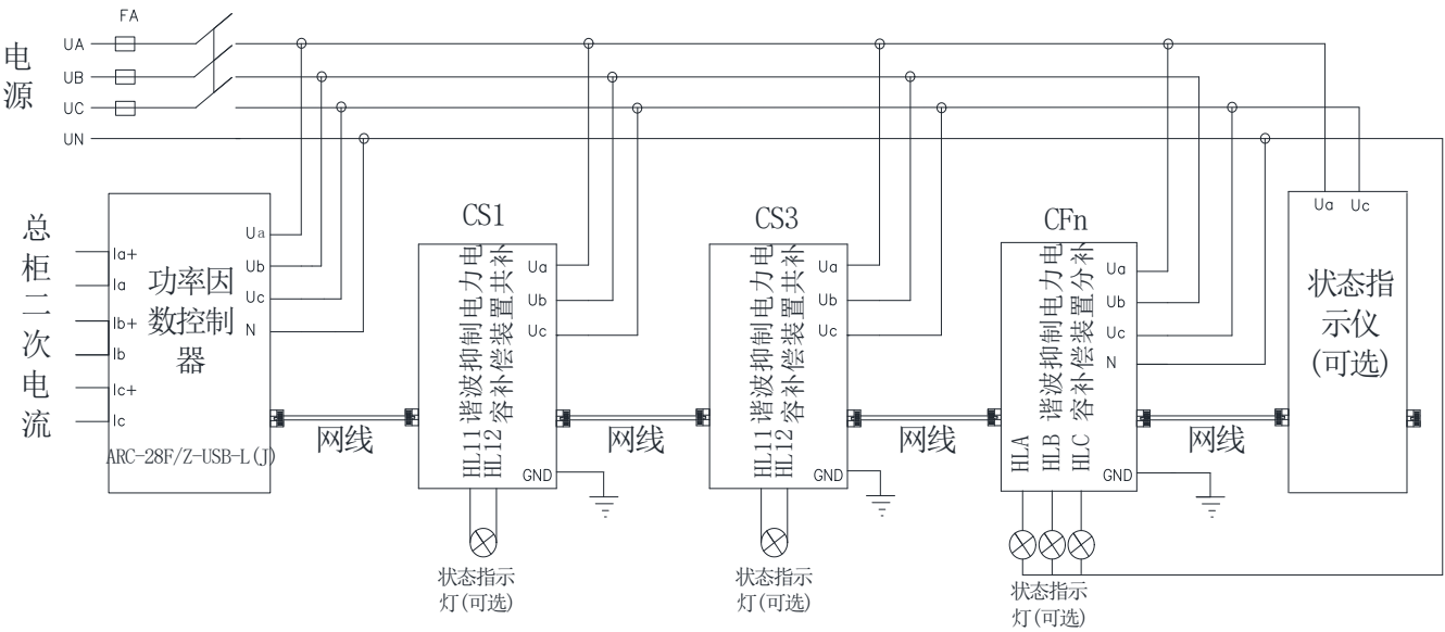
图 135 混补接线图
