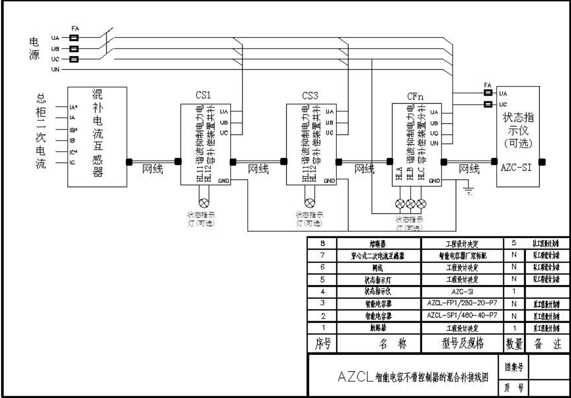
图 97 不带无功补偿控制器的混补接线图
