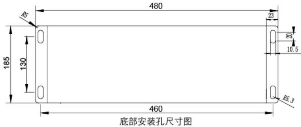
图 93 安装尺寸图
